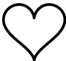
heart
